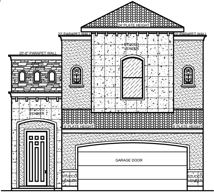
OPTION(B) SCALE: 1/4" = 1'-0"
